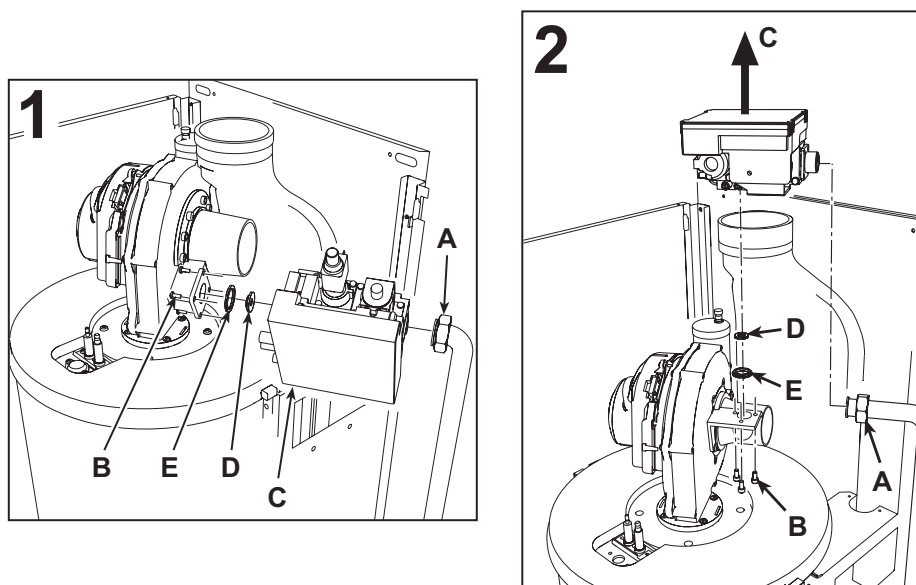
fig. 39 - Trasformazione gas
