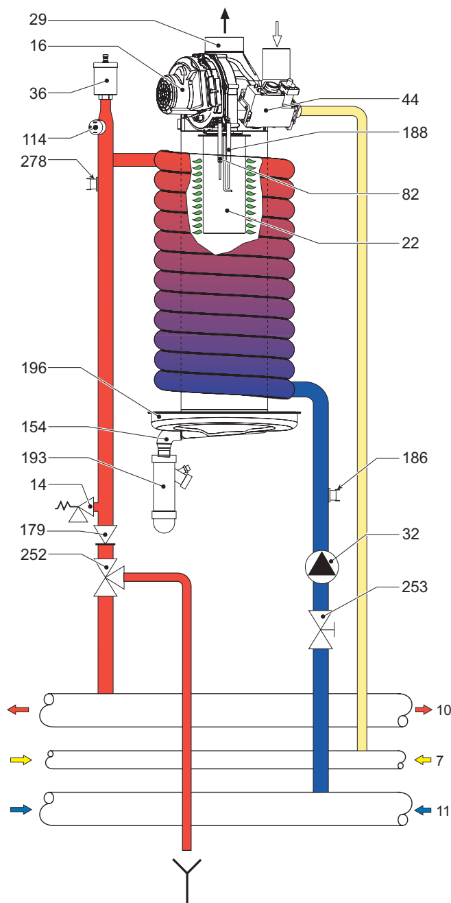
fig. 45 - Circuito idraulico modello ENERGY TOP B 80 - 125
