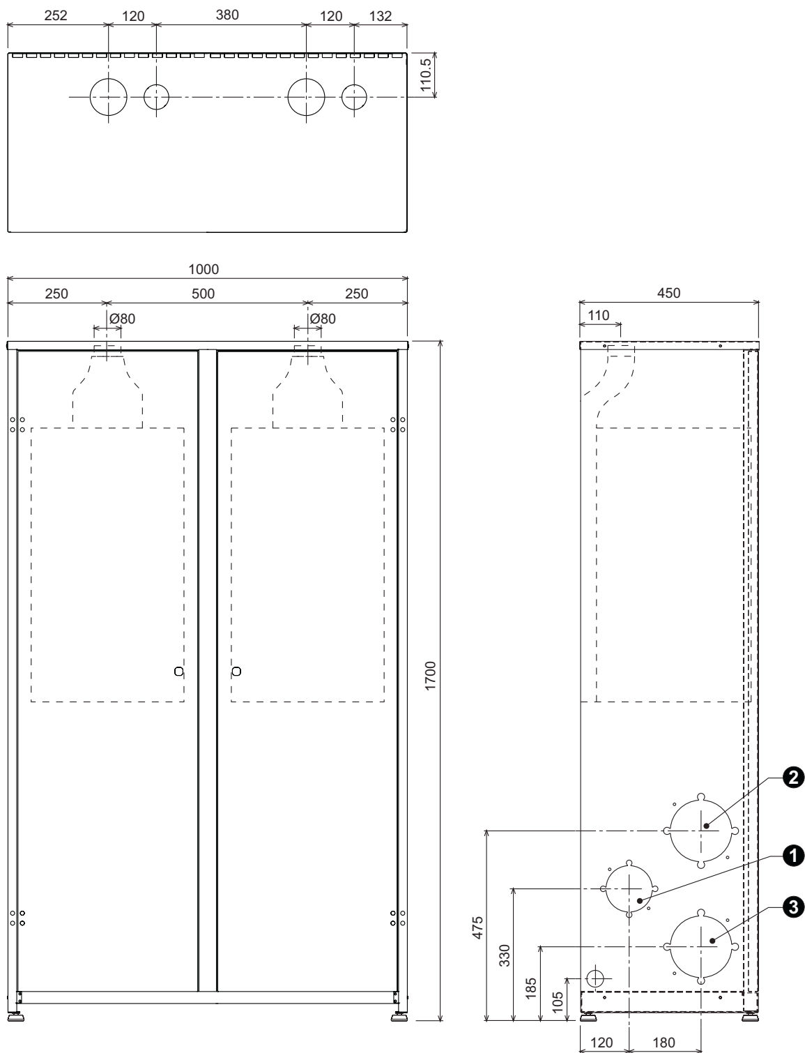
fig. 42 - Dimensione e attacchi modello ENERGY TOP B 160 - 250
