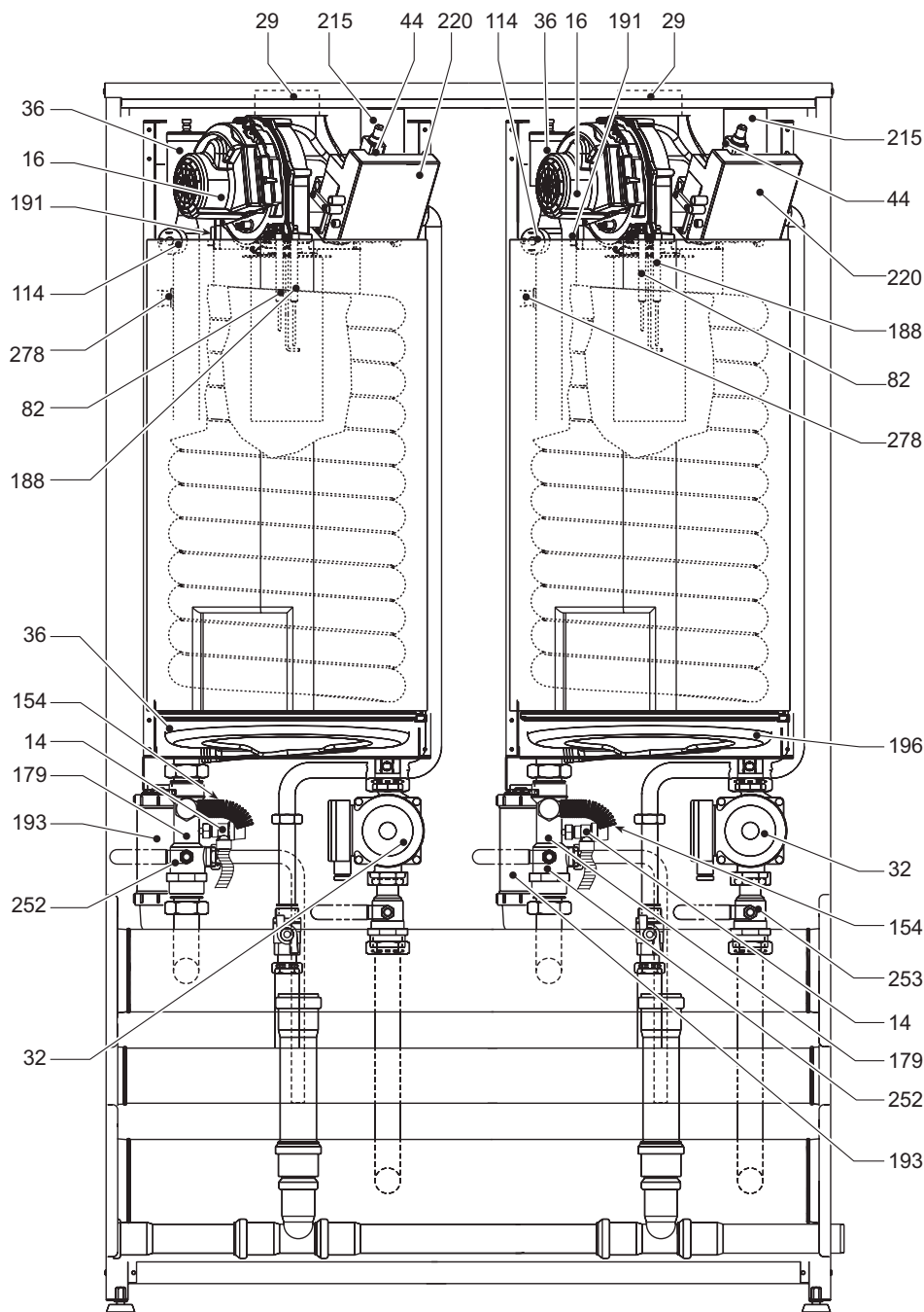
fig. 44 - Vista generale modello ENERGY TOP B 160 - 250
