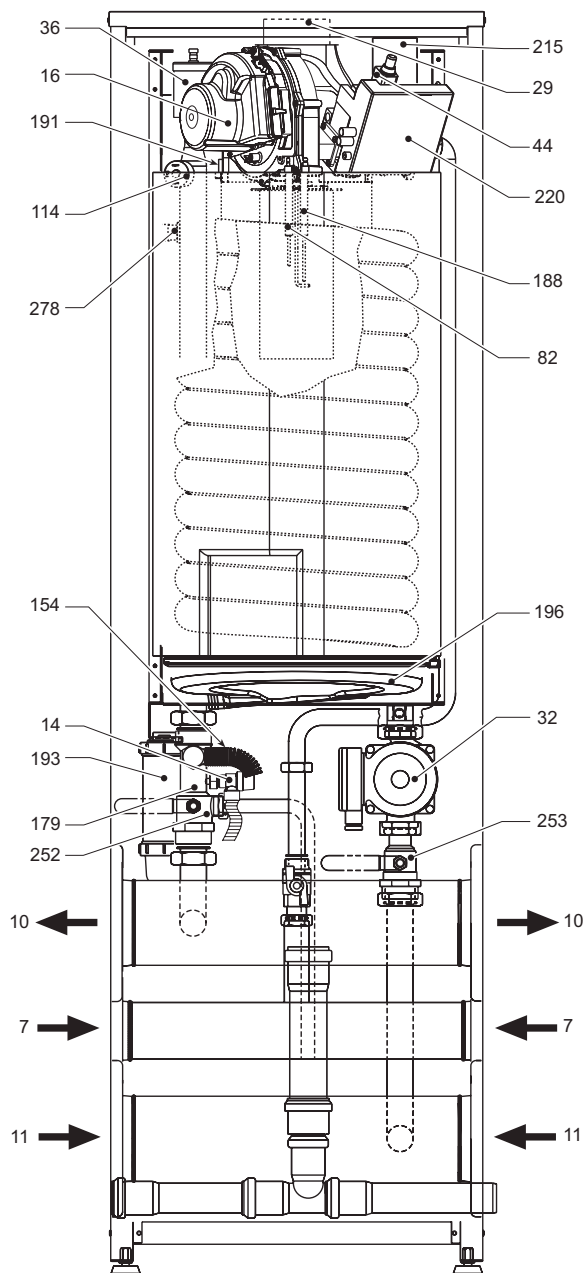
fig. 43 - Vista generale modello ENERGY TOP B 80 - 125
