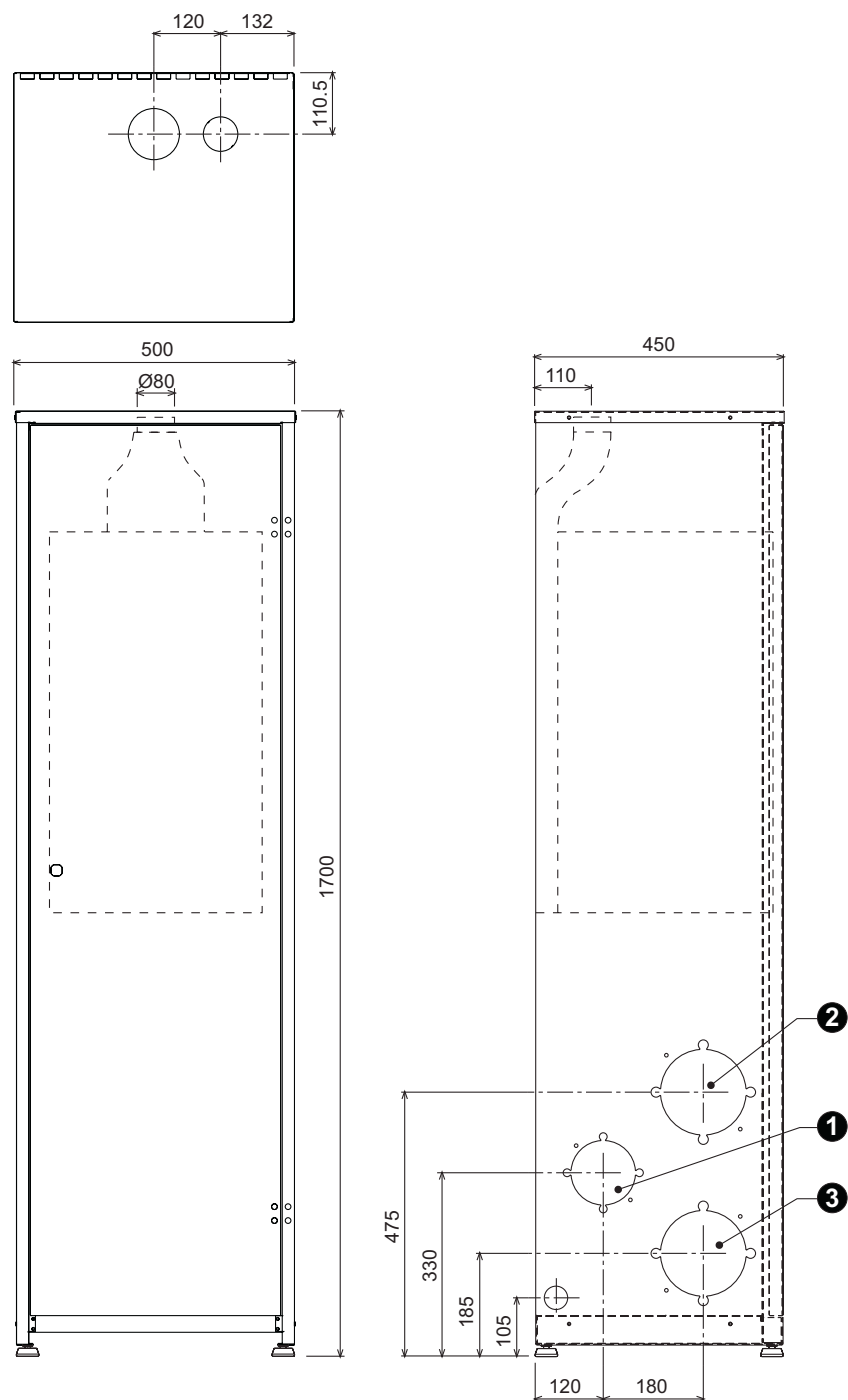
fig. 41 - Dimensioni e attacchi modello ENERGY TOP B 80 - 125
