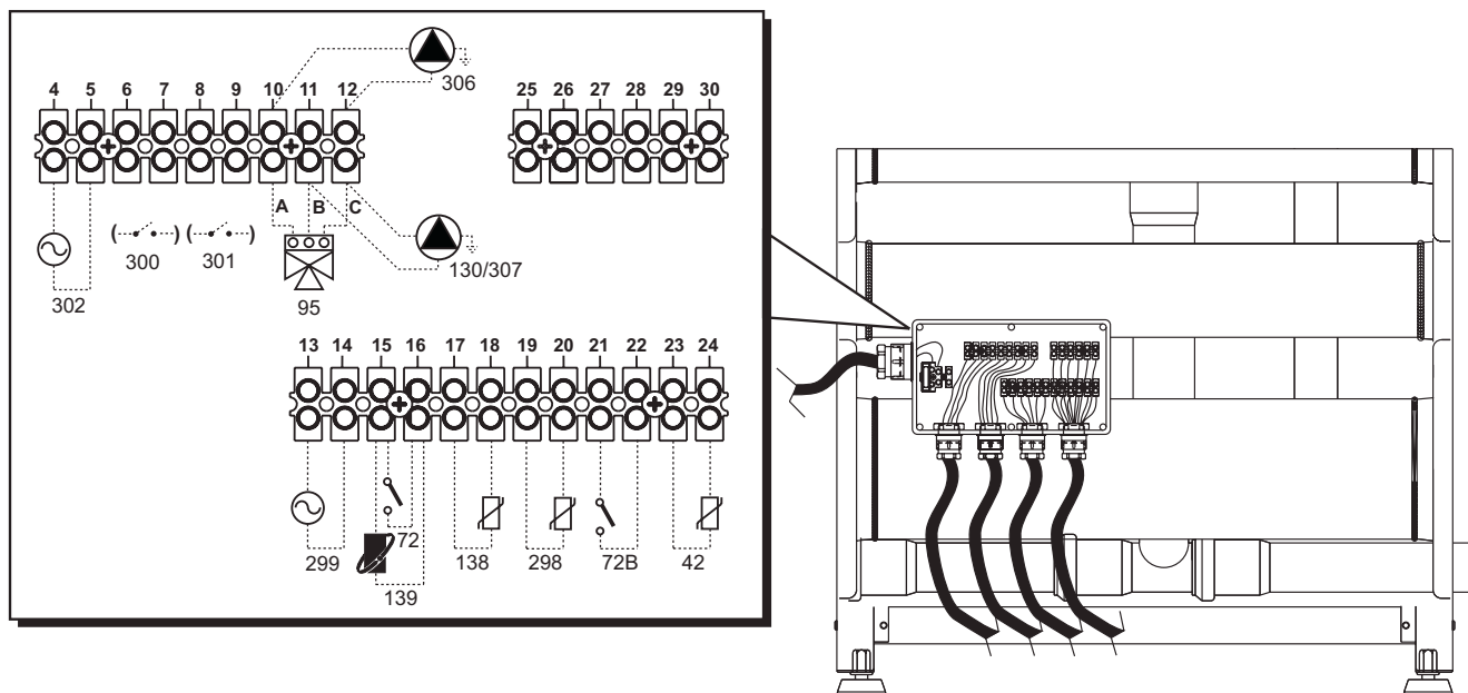
fig. 30 - Morsetteria elettrica
