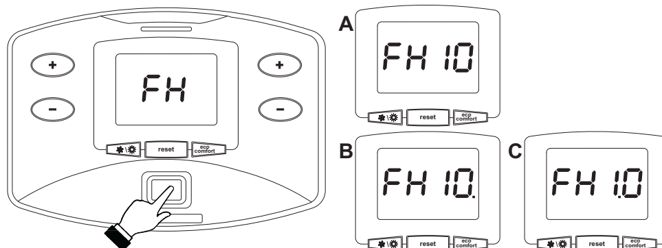
fig. 4 - Accensione caldaia
