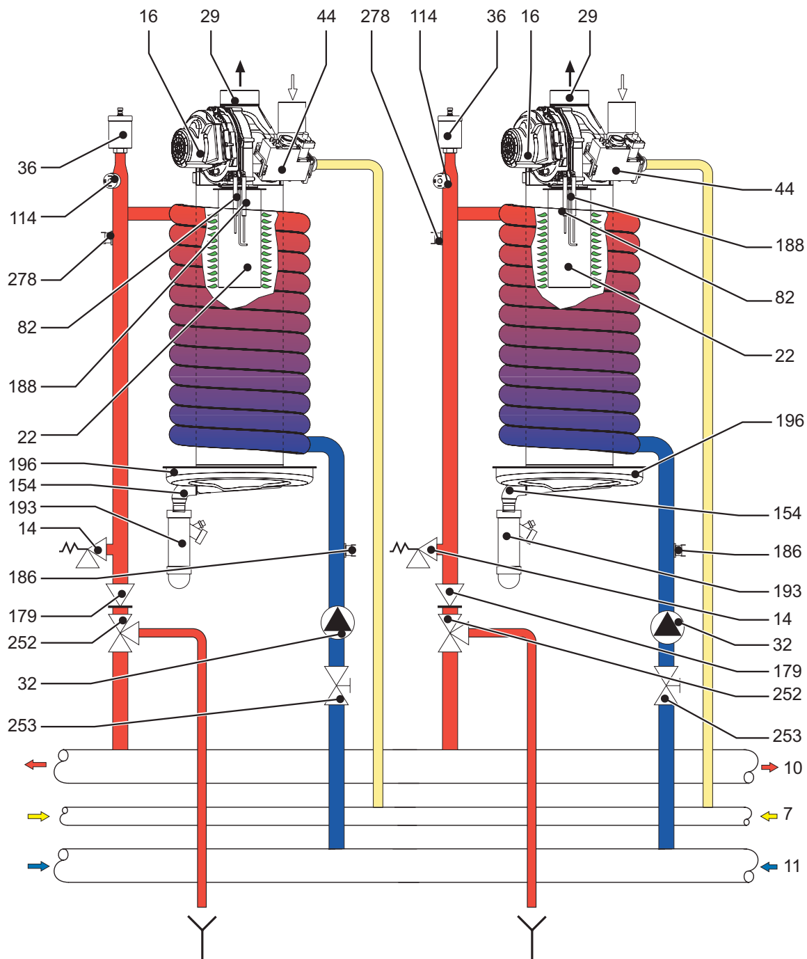
fig. 46 - Circuito idraulico modello ENERGY TOP B 160 - 250
